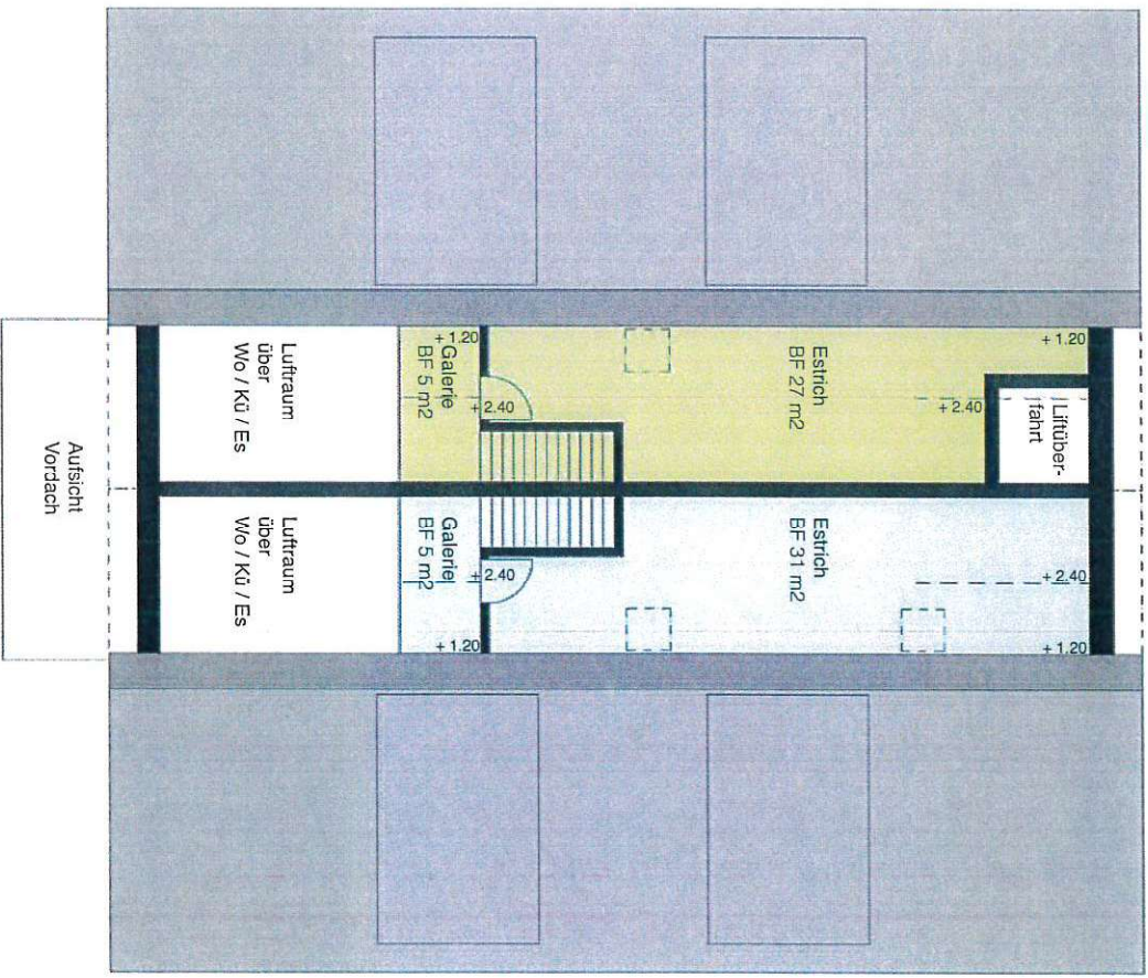
Dachgeschoss 1:100
