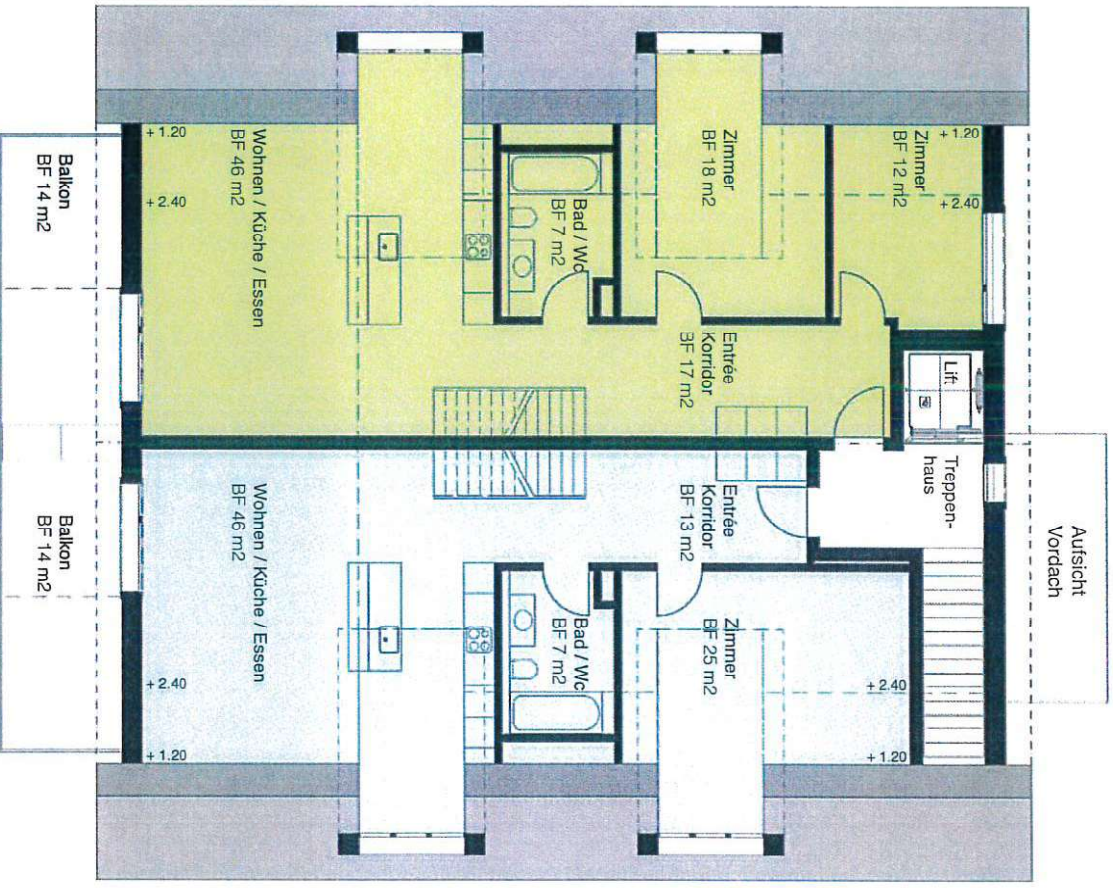
Obergeschoss 1:100
